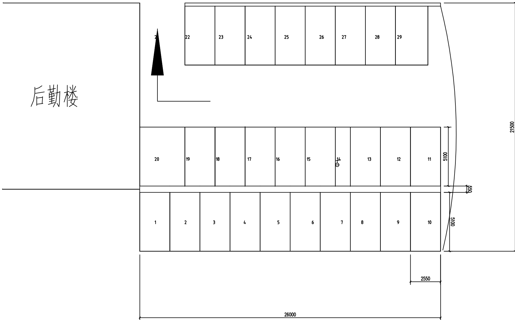
后勤楼侧空地改建临时停车方案示意图
